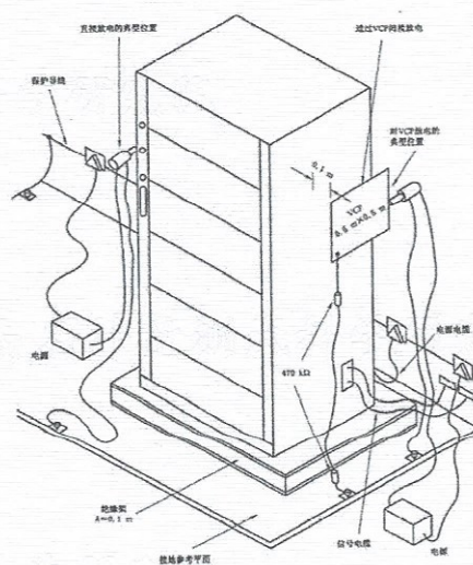
布置示意图
