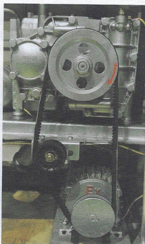
油泵（含油气分离器）
