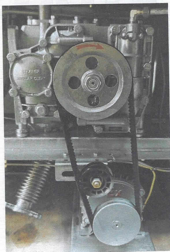
油泵（含油气分离器）
