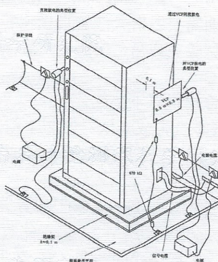
布置示意图
