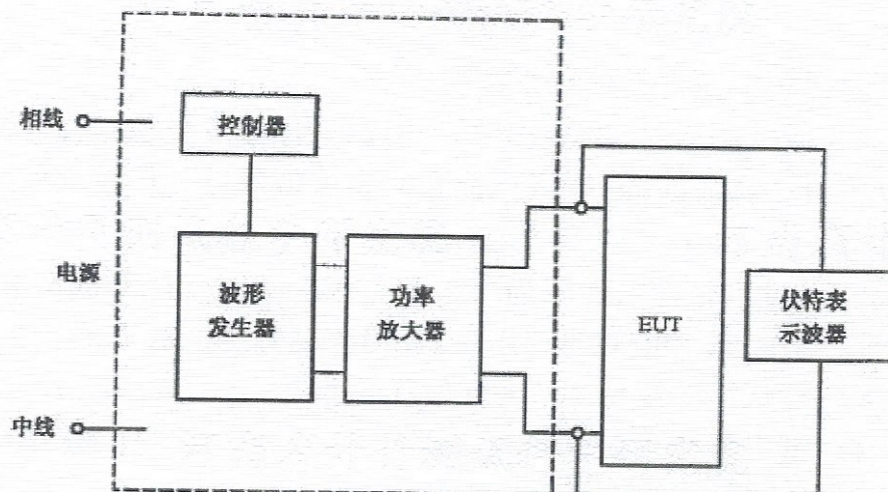
布置示意图
