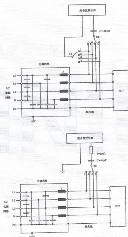
布置示意图
