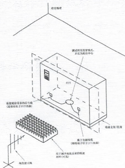
布置示意图
