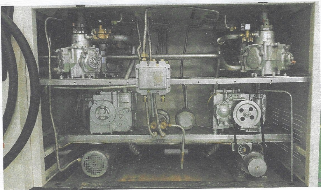
下部结构
