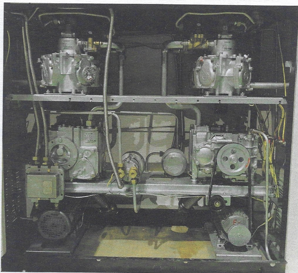
下部结构
