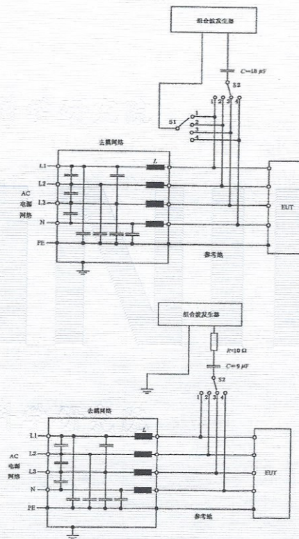
布置示意图
