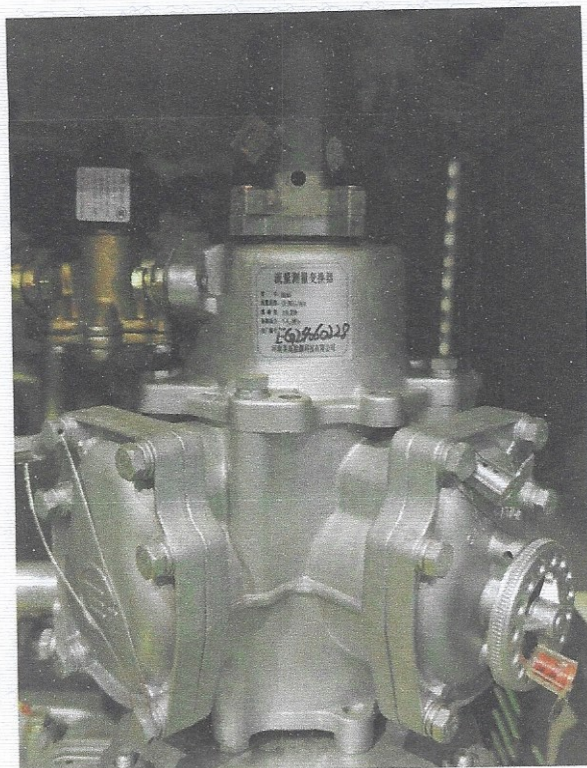
流量测量变换器
